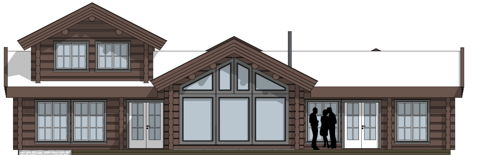
1:100 Fasade Vest
